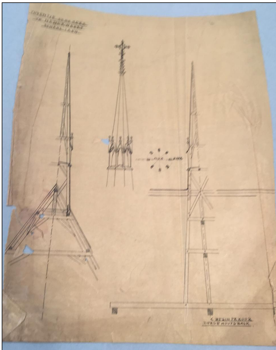
Fig. 7. Ontwerptekening van de nieuwe Angelustoren, ca. 1900 door architect Cuijpers. Het Nieuwe Instituut, CUBA Cuijpers Bureau-Archief 110381098, foto Aagje Gosliga.
