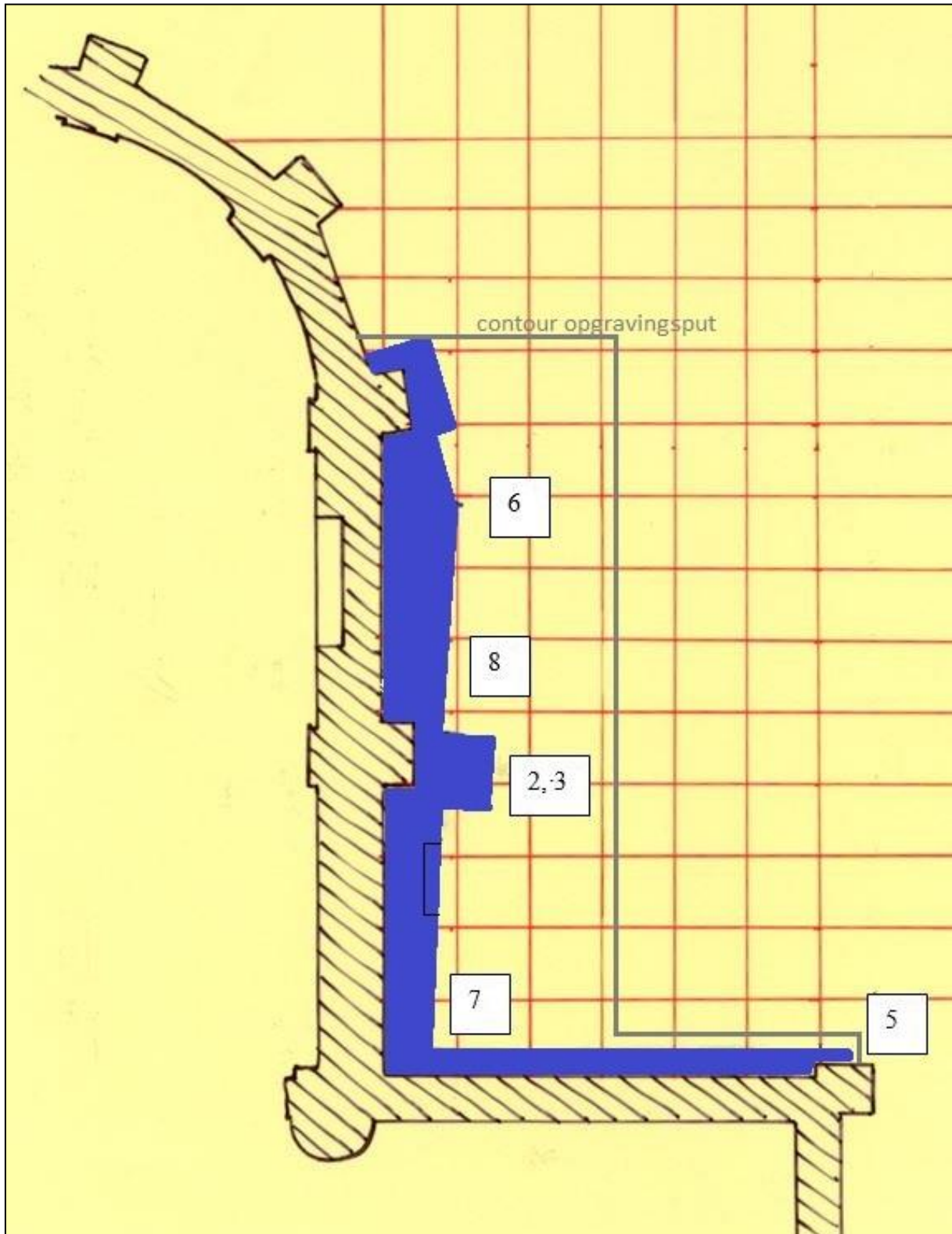
Figuur 1. Plattegrond van de aangetroffen sporen. In zwarte arcering het opgaande werk uit 1844. In blauw de contour van de ondergrondse, oudere funderingsspooren. Het rode raster meet 1x1 m. De grijze lijn is de contour van de opgravingsput. Het zwarte rechthoekje in de blauwe zone is de aangetroffen rollaag. De nummers verwijzen naar de figurnummers van de foto's (zie hierna).
