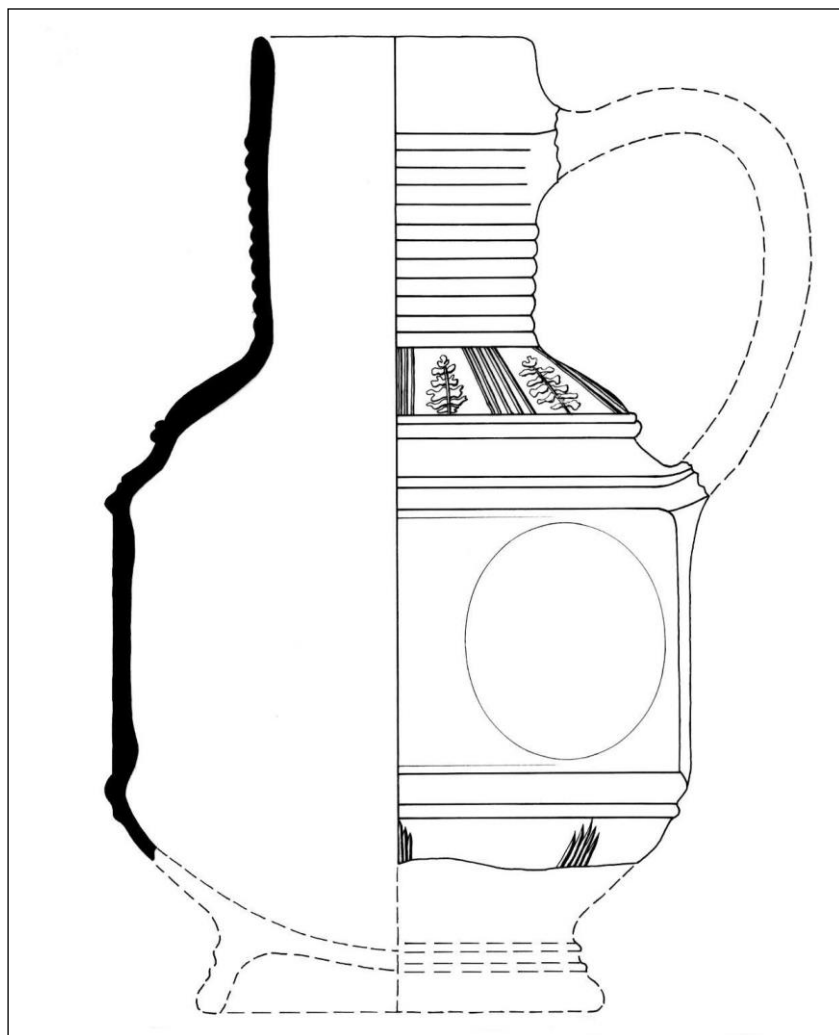
Figuur 3. De Raerense cilinderkruik van Oelemarkt 11. Schaal 2:1. De fries is apart afgebeeld. Tekening: Alfons Bruekers.
